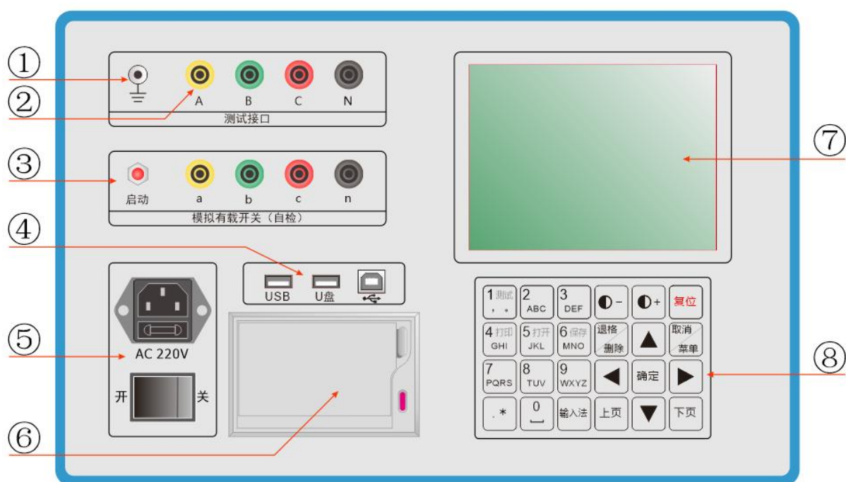
图 6.1 面板图
